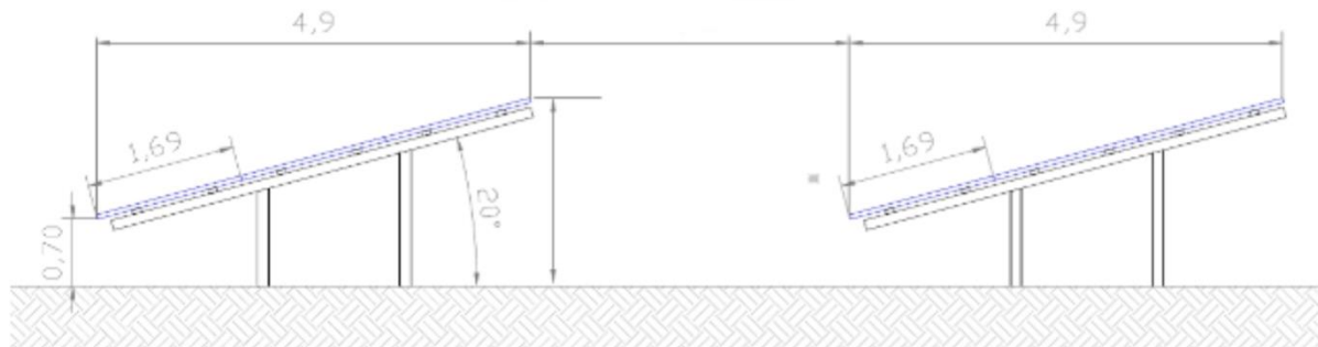
Rysunek 4. Rzut na przykładową konstrukcję stołów z panelami fotowoltaicznymi (rozwiązanie typowe, najczęściej stosowane).
